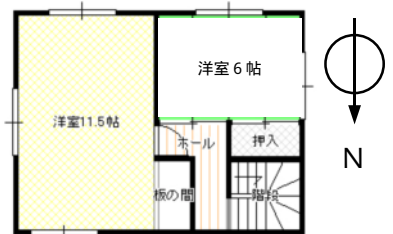
2階平面図 38.93㎡
