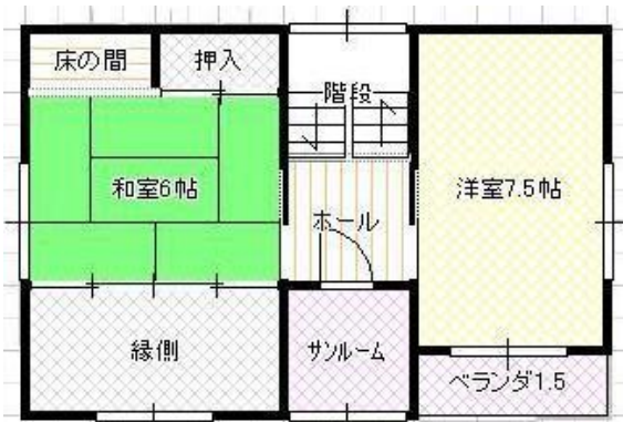
2階平面図
